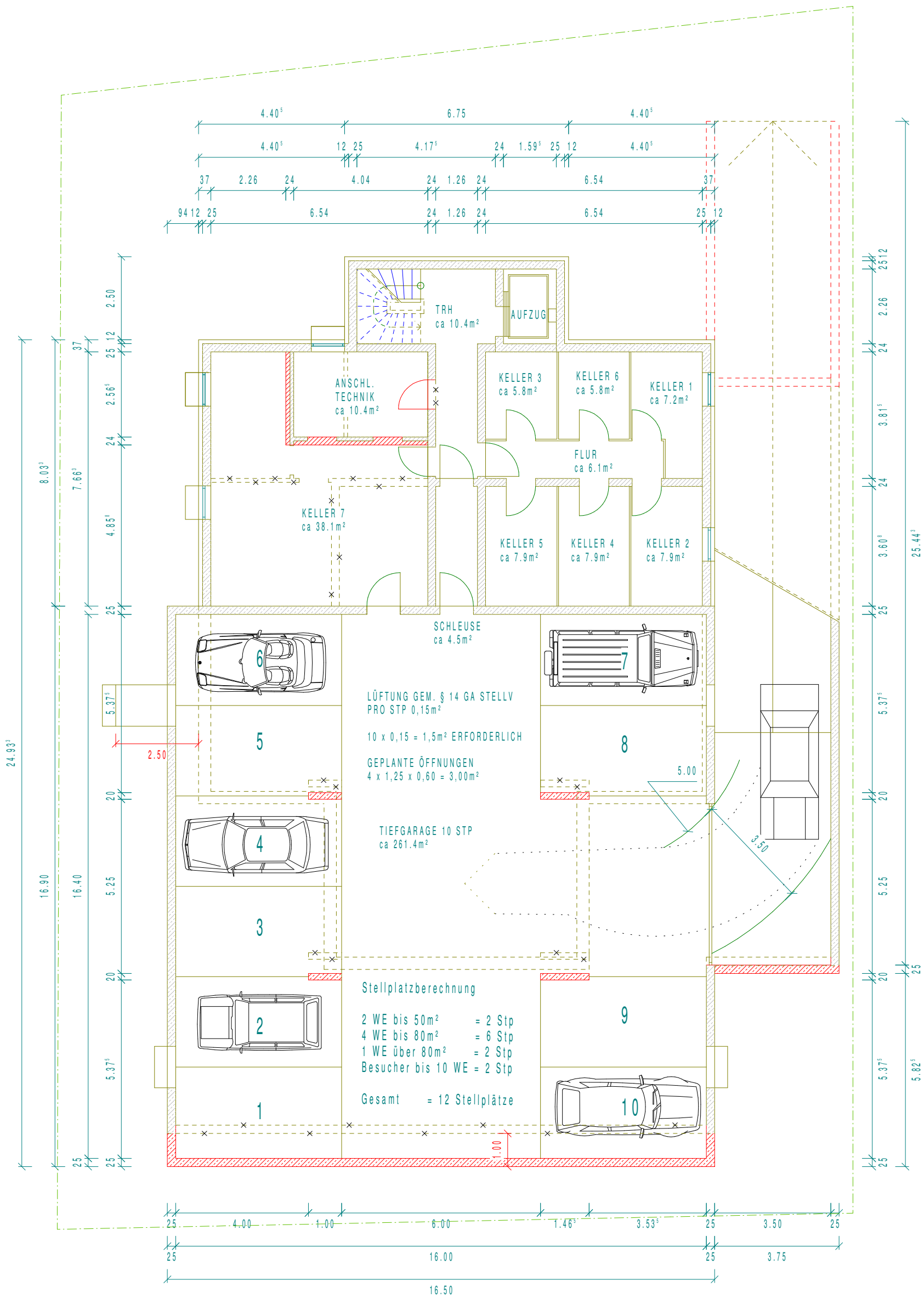
GRUNDRISS KG
